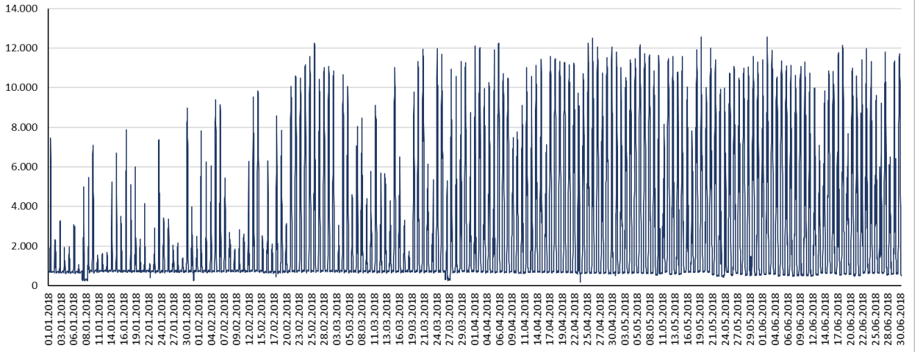
Einspeisekurve in die Netzebene 7 - 1. Halbjahr
