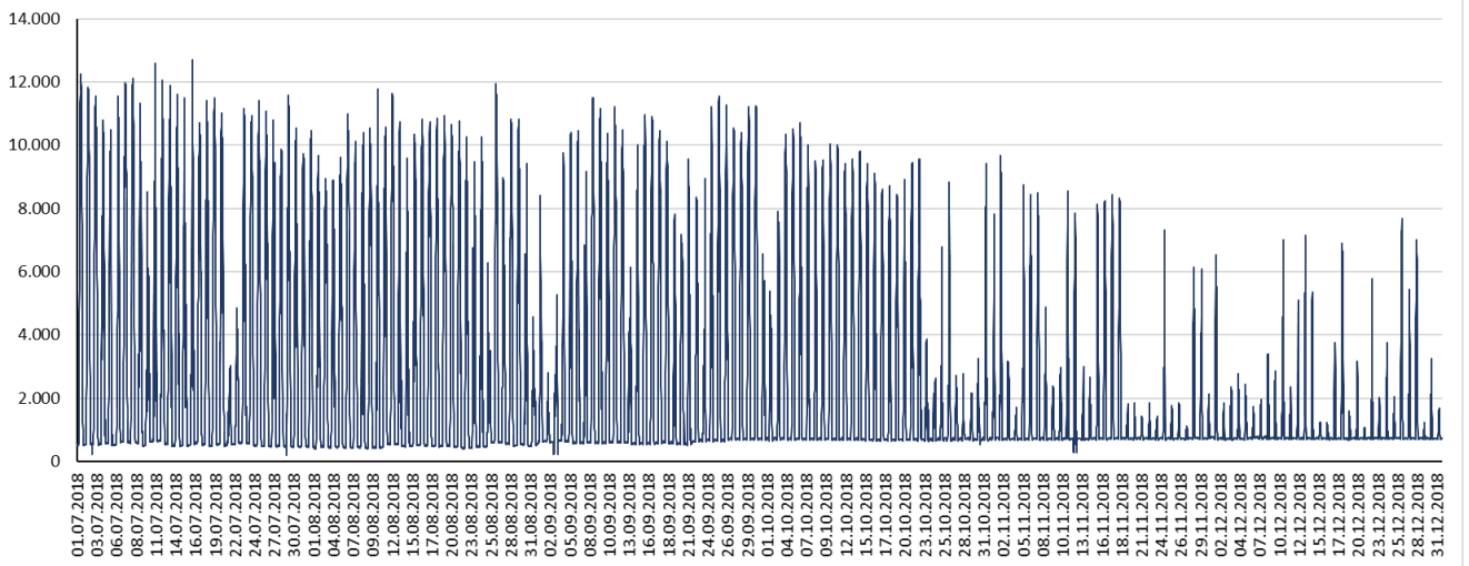
Einspeisekurve in die Netzebene 7 - 2. Halbjahr
