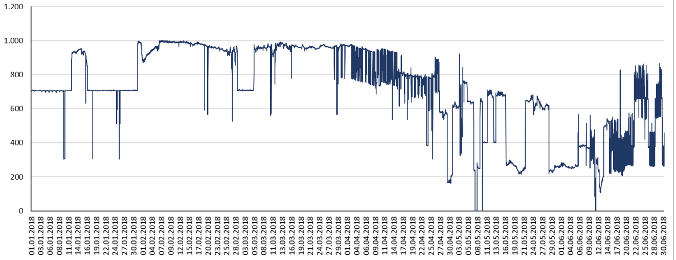
Einspeisekurve in die Netzebene 6 - 1. Halbjahr
