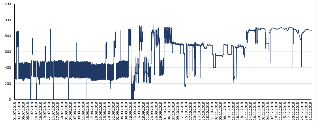
Einspeisekurve in die Netzebene 6 - 2. Halbjahr
