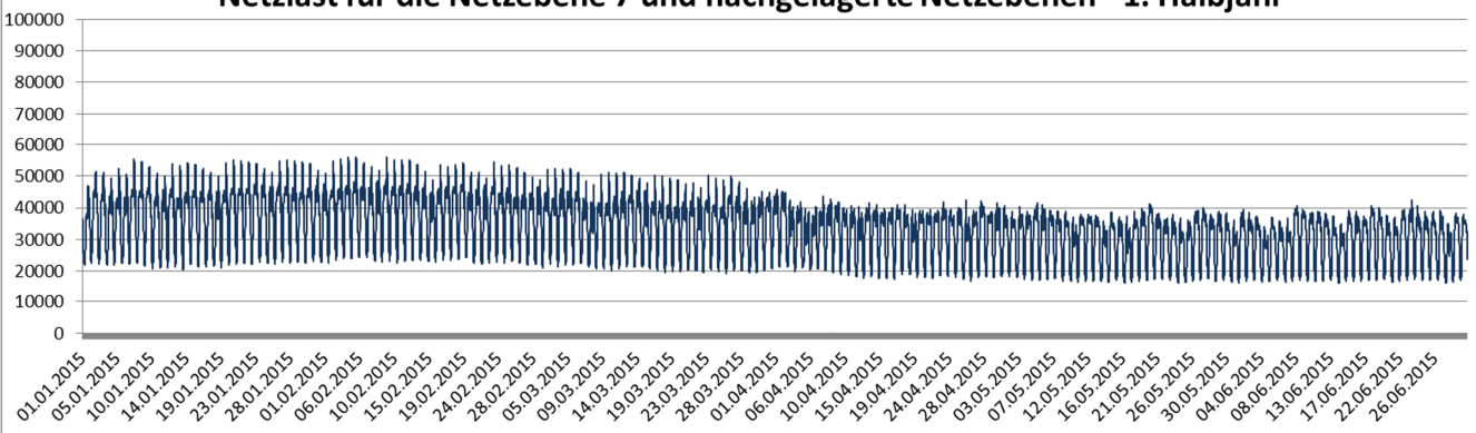
Netzlast für die Netzebene 7 und nachgelagerte Netzebenen - 1. Halbjahr
