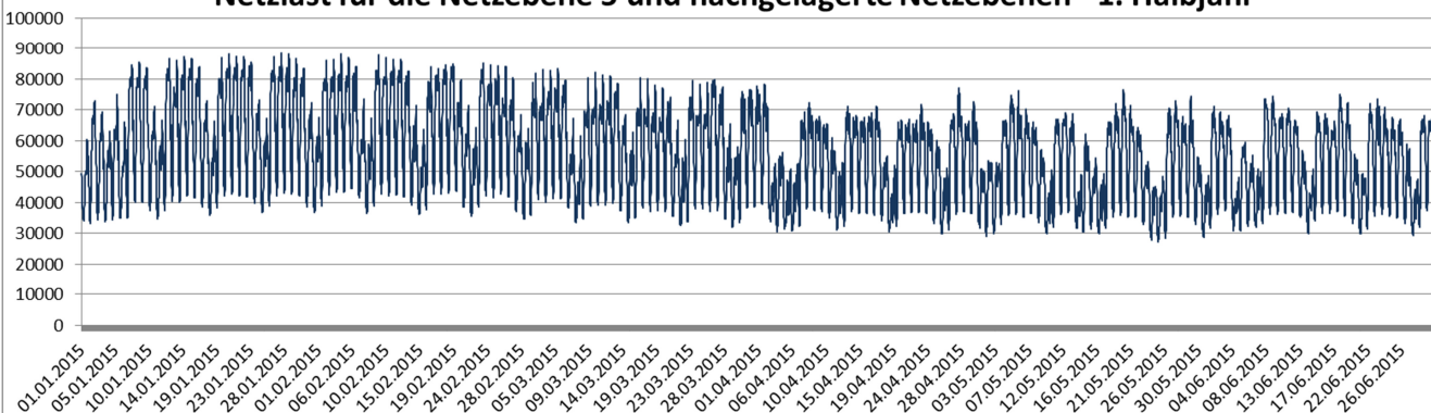
Netzlast für die Netzebene 5 und nachgelagerte Netzebenen - 1. Halbjahr
