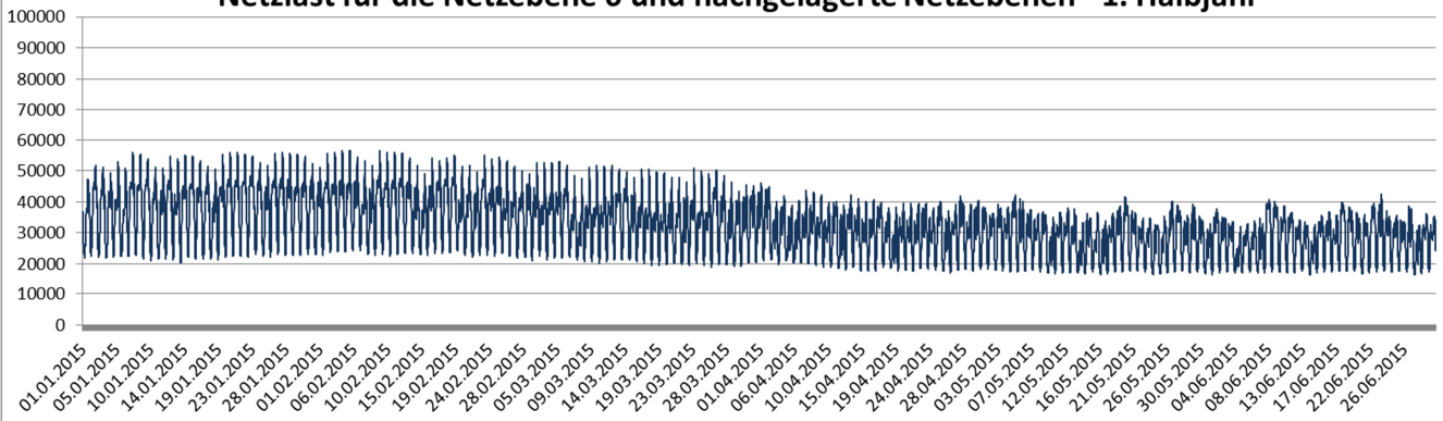
Netzlast für die Netzebene 6 und nachgelagerte Netzebenen - 1. Halbjahr
