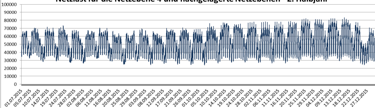
Netzlast für die Netzebene 4 und nachgelagerte Netzebenen - 2. Halbjahr
