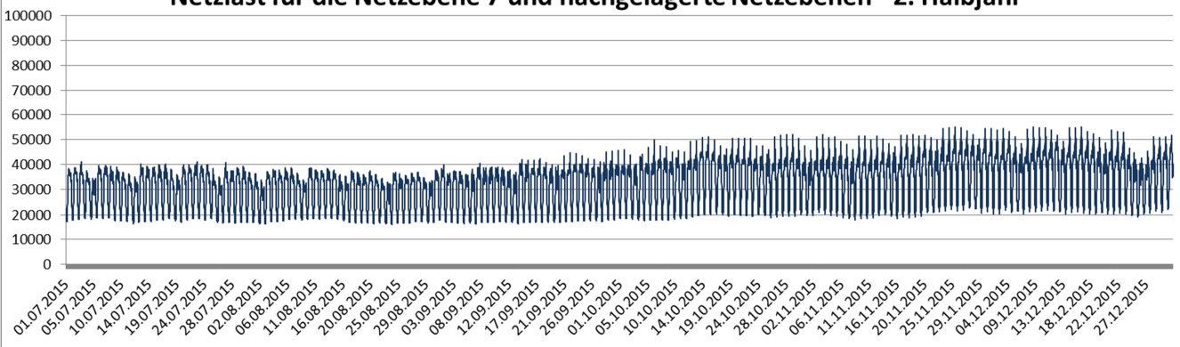
Netzlast für die Netzebene 7 und nachgelagerte Netzebenen - 2. Halbjahr
