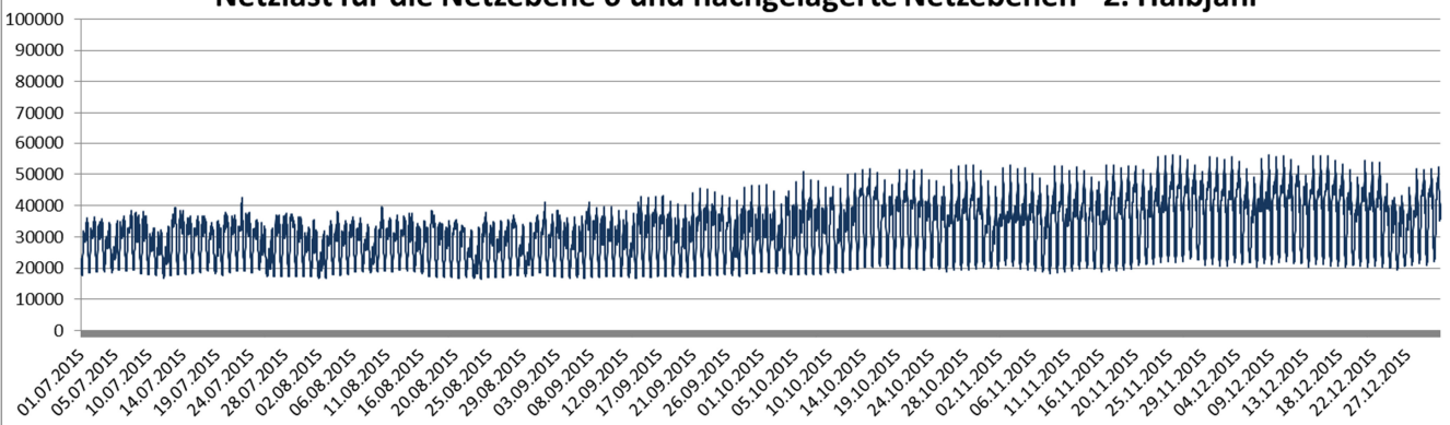
Netzlast für die Netzebene 6 und nachgelagerte Netzebenen - 2. Halbjahr
