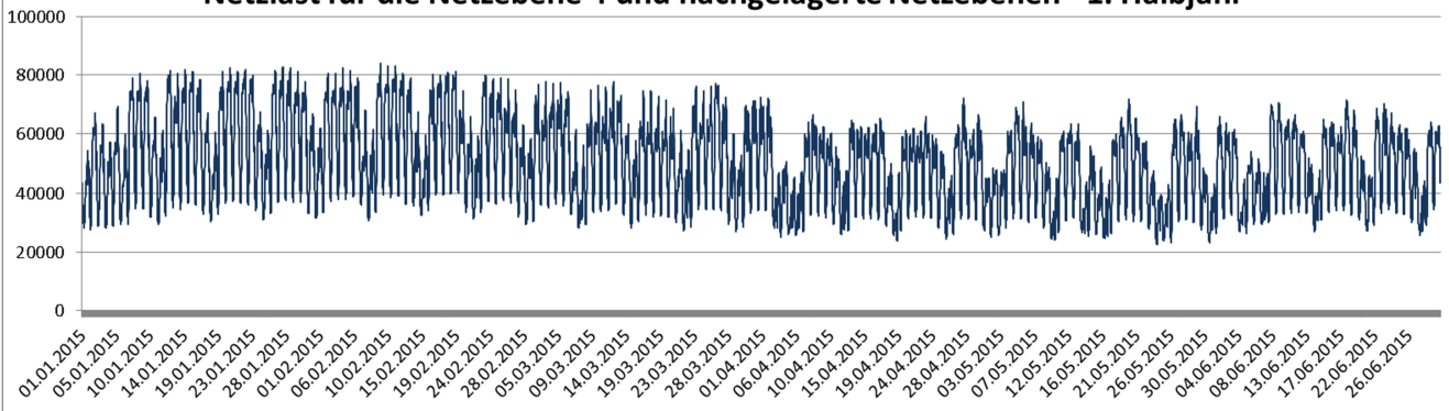
Netzlast für die Netzebene 4 und nachgelagerte Netzebenen - 1. Halbjahr
